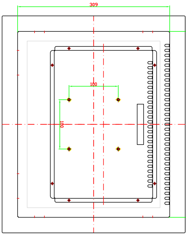
Achter-aanzicht:
